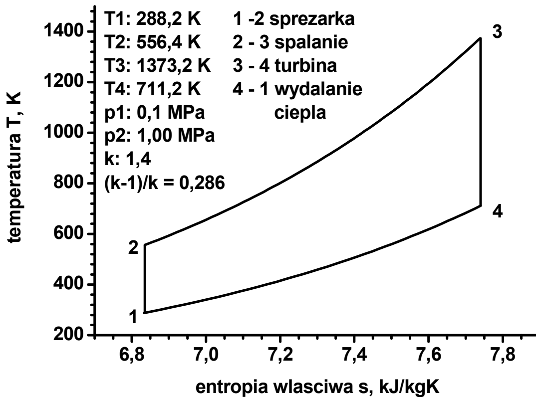
Cykl Braytona, diagram T, s
