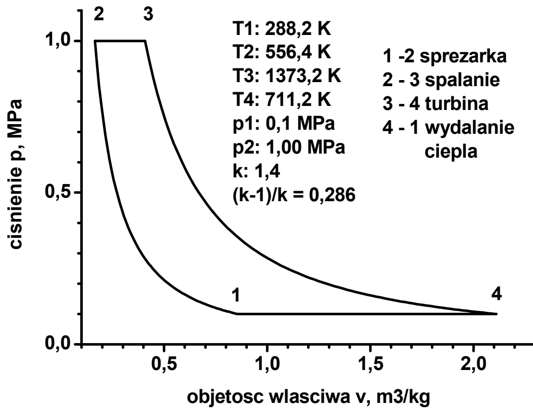
Cykl Braytona, diagram p, v
